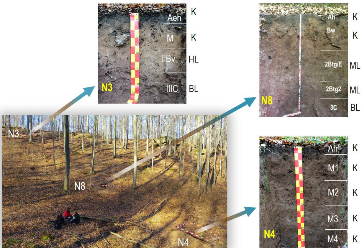
Abb. 1: Catena im Buntsandsteingebiet bei Ebergötzen, ca. 10 km östlich von Göttingen (Fotos: D. Sauer). K = Kolluvium, HL = Hauptlage, ML = Mittellage, BL = Basislage.
